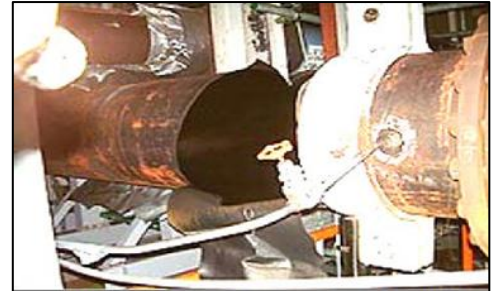
▲ 2004年8月美浜原発の復水管破裂
