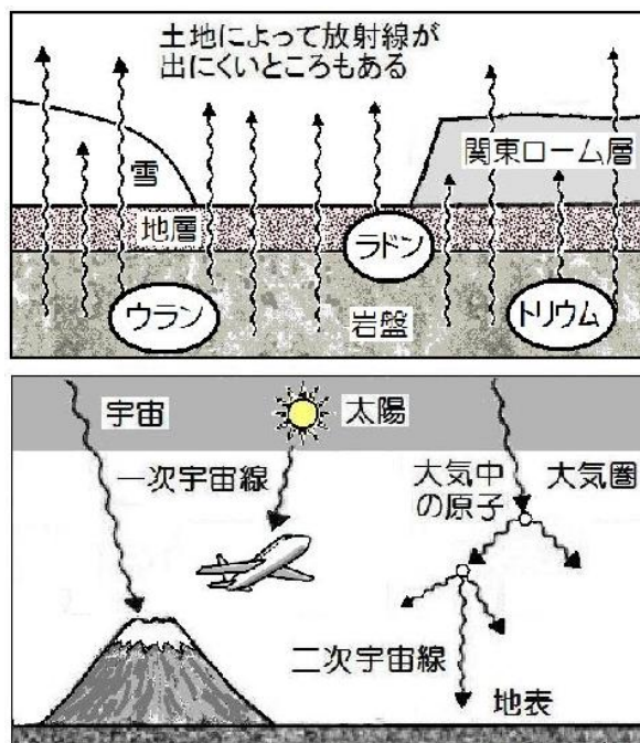
【地殻と宇宙から受ける自然放射線】
