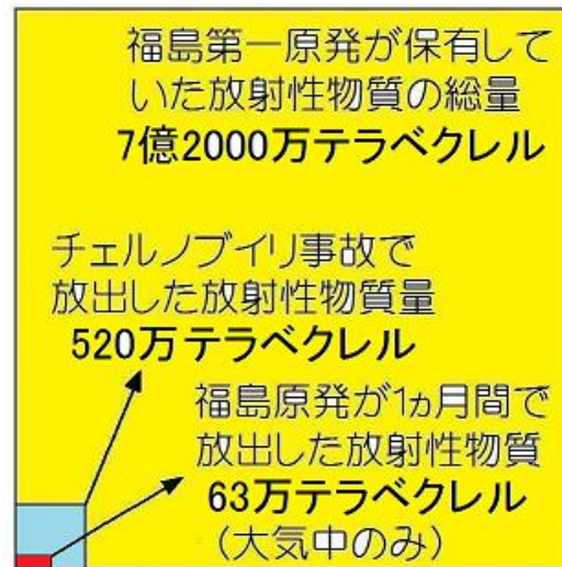
▲大気に流出した放射性物質量の比較
